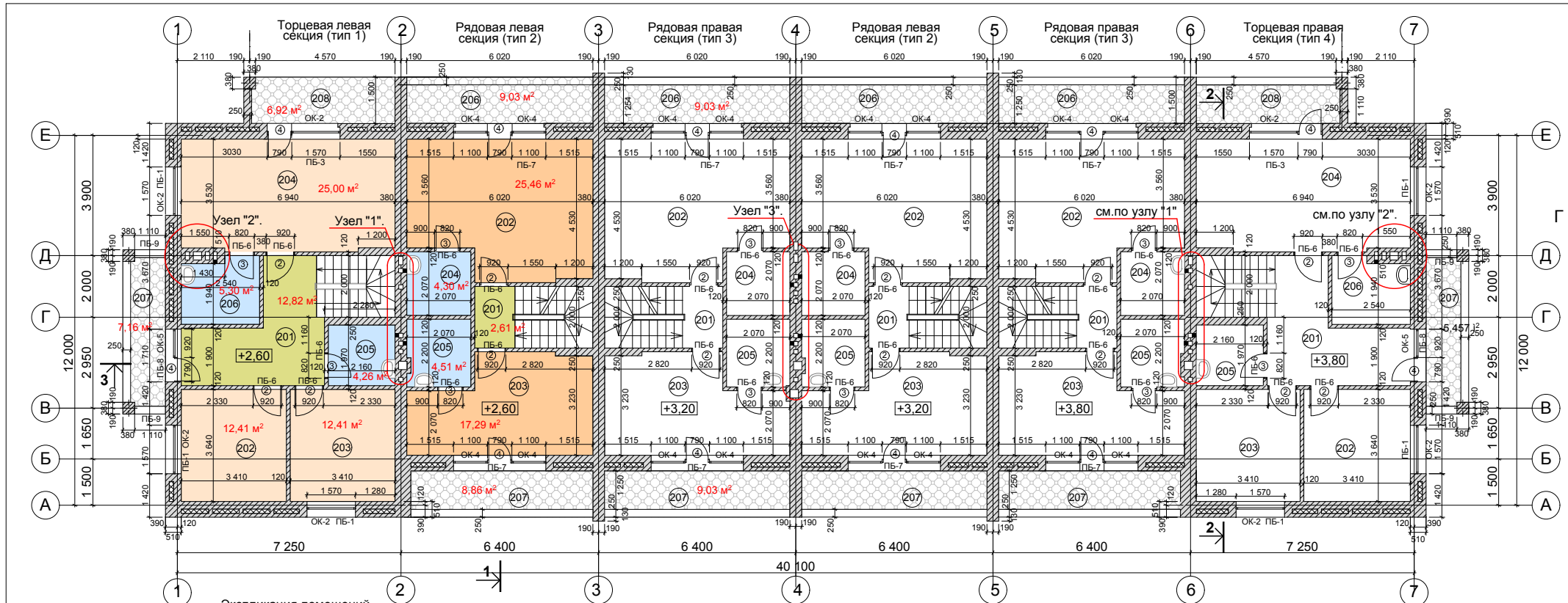
Экспликация помещений рядовой секции (тип 2)
