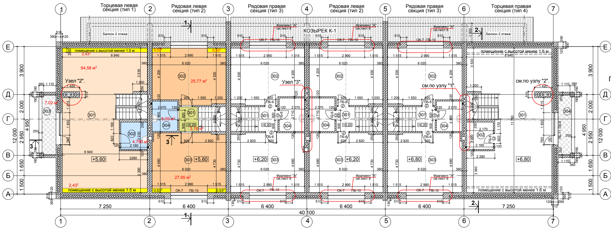
Экспликация помещений торцевой секции (тип 1, 4)
